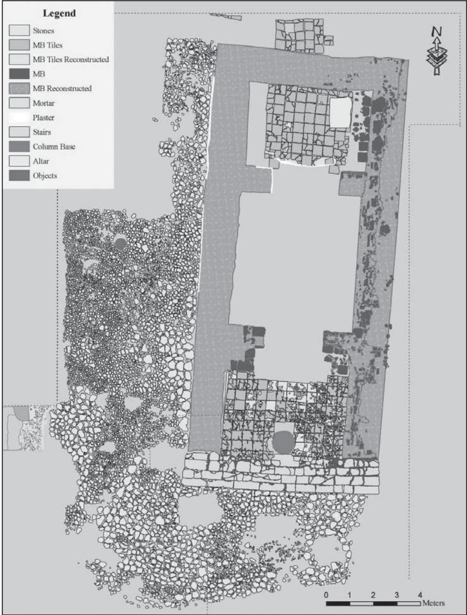
Resim 5: Alan 2'deki tapınak kompleksinin planı.
