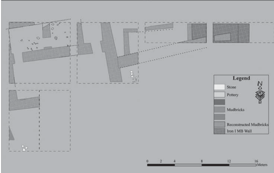
Resim 15: Alan 5'teki Demir Çağı II'ye tarihlenen avlulu 'idarî bina'.
