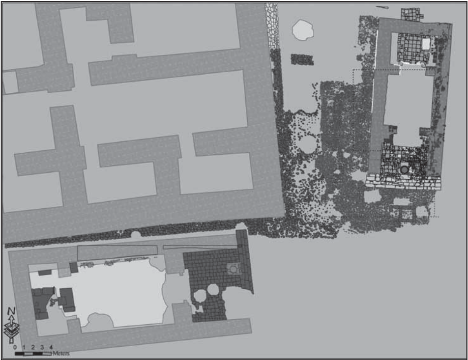
Resim 13: İki tapınak ve anıtsal yapıyı içeren 'dinî kompleks'in planı.
